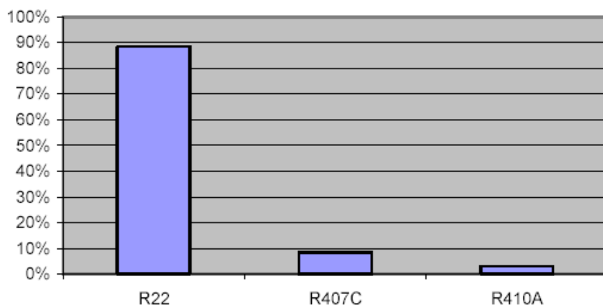
Figur 3.4 Arbeidsmedier i 608 Eurovent-testede varmepumper (Nowacki, 2002).
