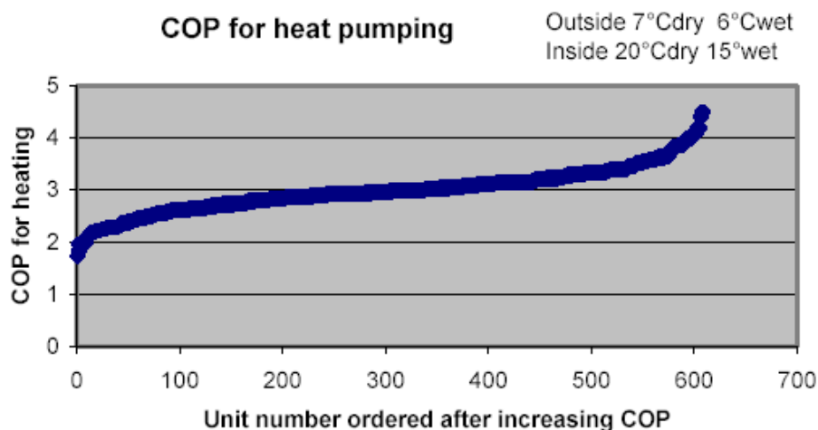
Figur 3.12 Varmefaktor for 608 varmepumper testet ved Eurovent (Nowacki, 2002).
