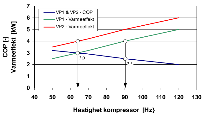
Figur 4.3 Eksempel på dellastkarakteristikk for to luft/luft-varmepumper.
