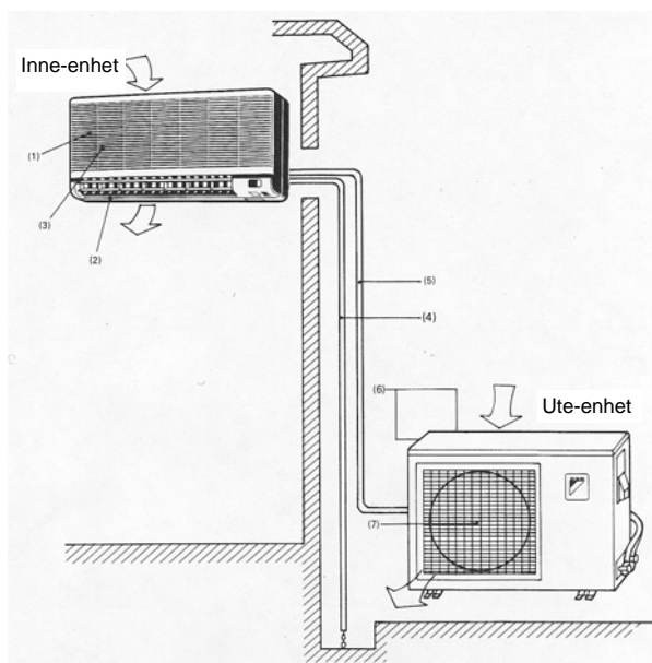
Figur 3.1 Luft/luft-varmepumpe for enebolig (split-anlegg).
