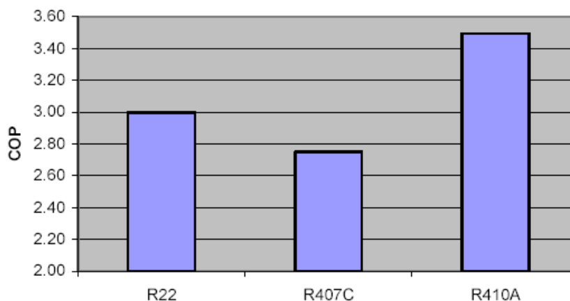
Figur 3.15 Varmefaktor for ulike arbeidsmedier (Nowacki, 2002).
