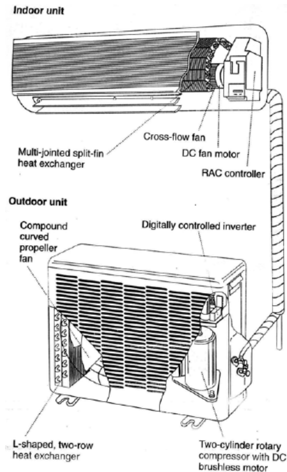
Figur 3.5 Typisk utforming av en luft/luft-varmepumpe (Nowacki, 2002).
